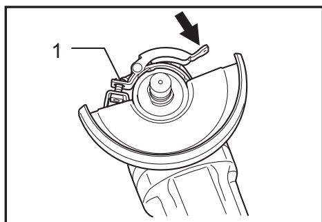
► 1. Tornillo
