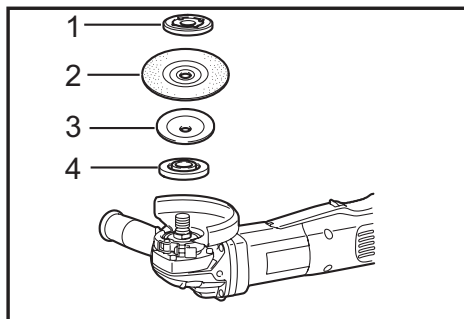
► 1. Contre-écrou 2. Meule flexible 3. Tampon d'apoint 4. Bague interne
